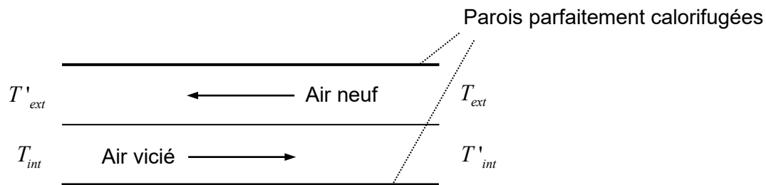
Figure 3 - Échangeur thermique
