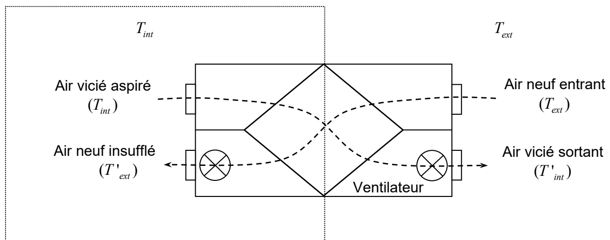
Figure 2 - Schéma de principe d'une VMC double flux
